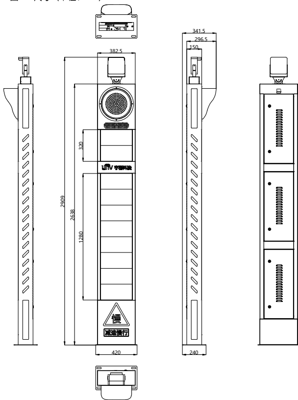
图2-2 尺寸 (单位: mm)
