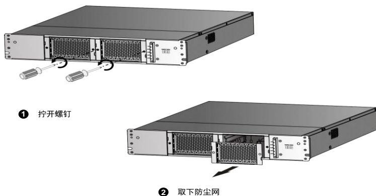
图2-3 拆卸防尘网
