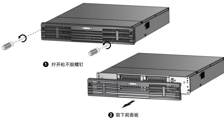
图2-3 拆卸防尘网
