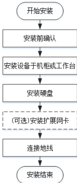
图2-1 安装流程图
